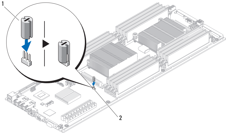
Abbildung 1. Installieren des Gummi-Jumpers
